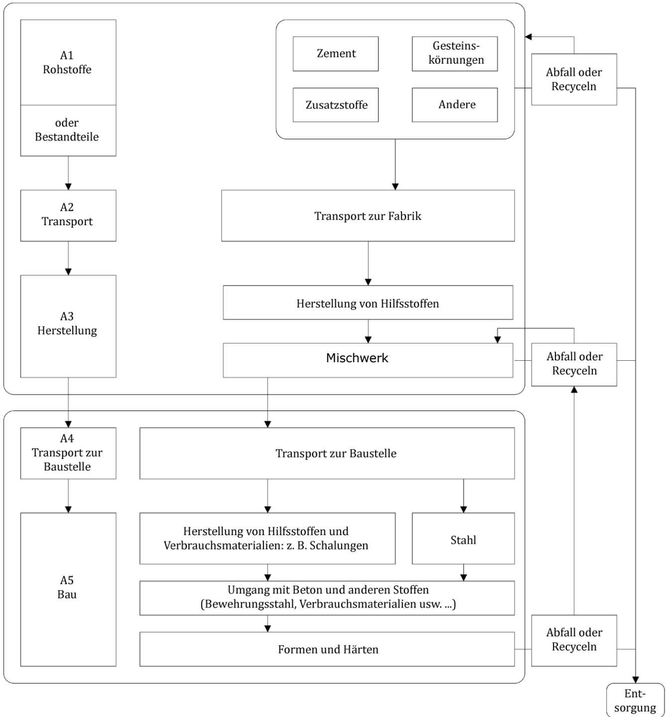
Abbildung 1: Systemgrenzen A1 - A5 für Transport- und Lieferbeton (ähnliche Produktionscharakteristika) [7]
